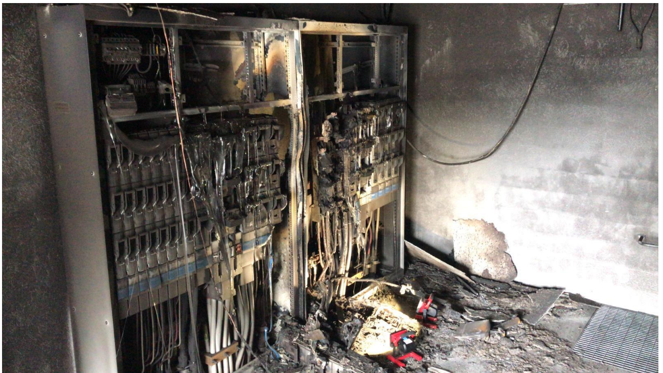
Durch den Brand zerstörte Niederspannungsverteilungen in der Trafostation Befang/Trogen von der SAK.
